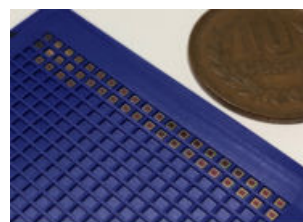
図2: 65nm CMOS プロセスの試作チップ
