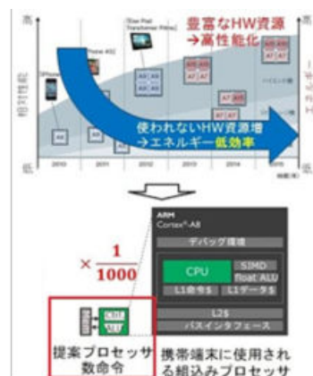
図1: 近年の組込みプロセッサの傾向(上)と本研究室で開発している超小型プロセッサ(下)
