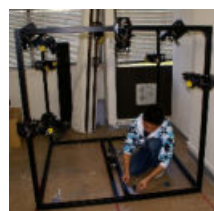
図2 多視点画像の計測
