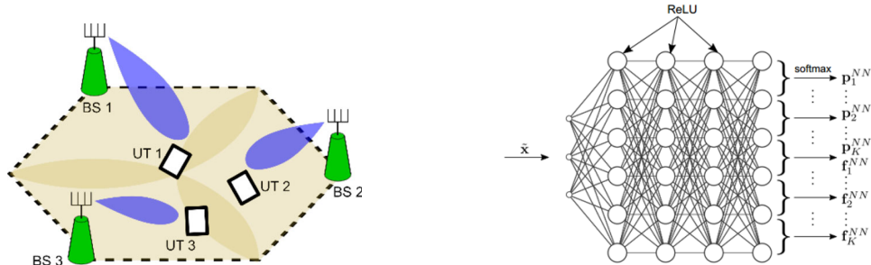
図 2. BS における送信ビームと送信電力制御 図 3. Deep Neural Network の構成例
