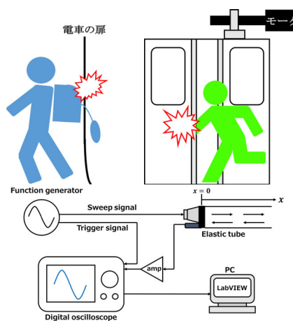
図5：戸挟みおよび検出システム
